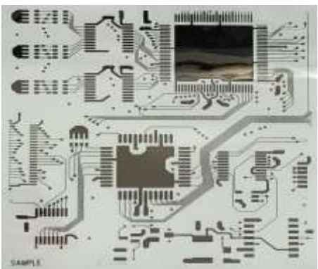
■アンカーコート処理したフィルムに銀ナノインクで印刷した回路図
